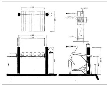
デザイン断面図
