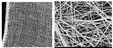
図2 ガーゼ(左)、3層構造のSMS不織布(右)
